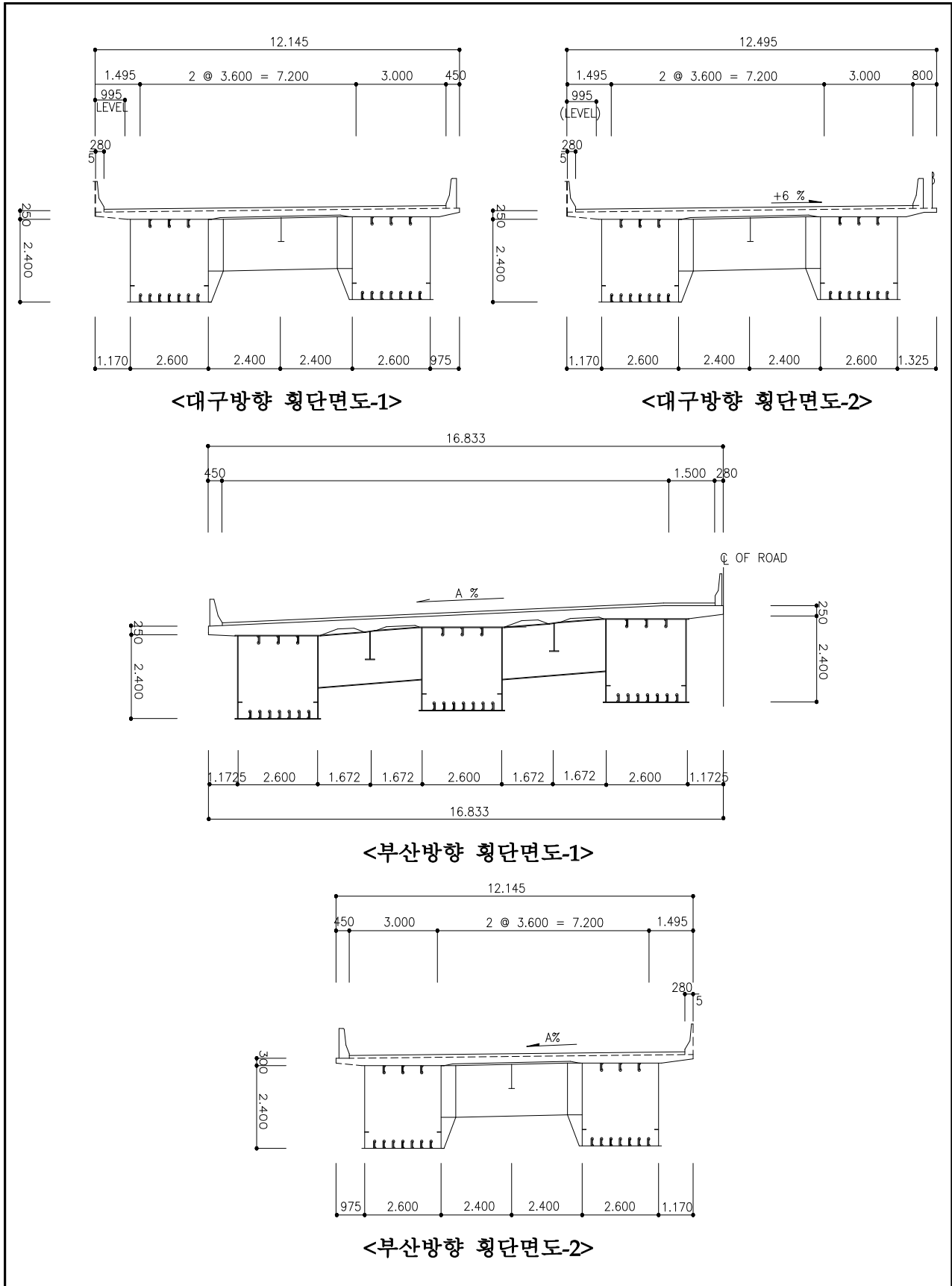
【그림 1.4.2】 청도1교 횡단면도
